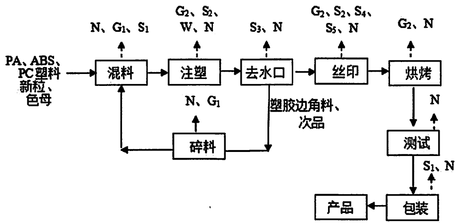
图 2-4 电池包、线扣套生产工艺流程图
