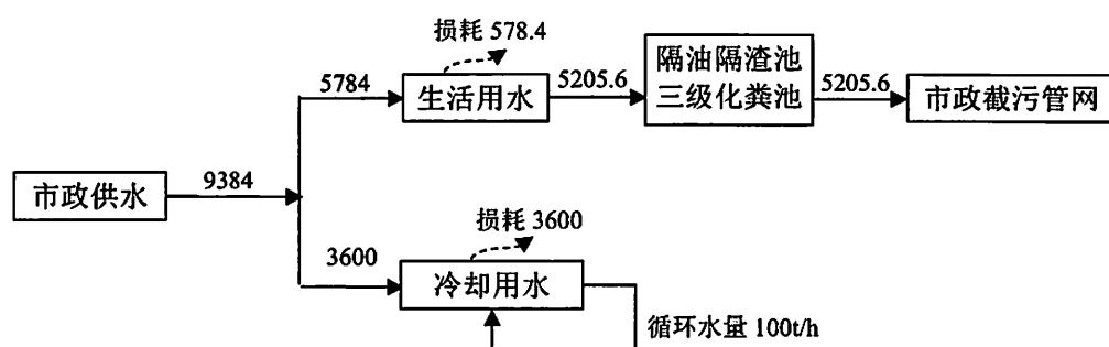
图 2-3 项目水平衡图（单位 t/a）
