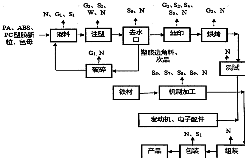
图 2-5 割草机生产工艺流程图
