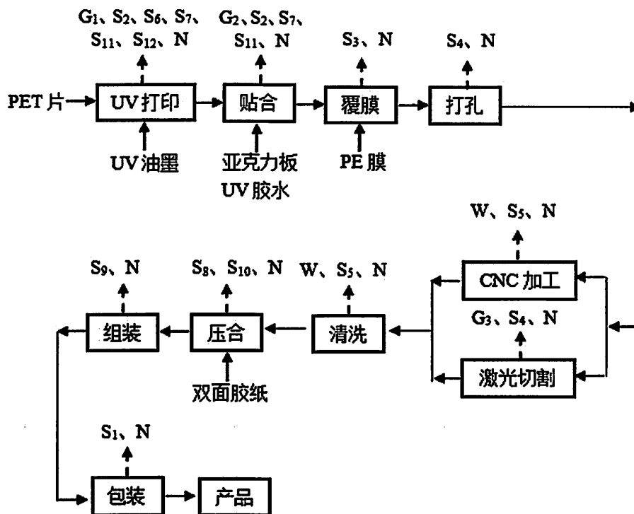
图 2-4 亚克力玩具摆件生产工艺流程图
